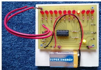
3. Binär-Zähler: Der Zähler hat eine etwas komischere Art zu zählen. Er zählt langsam und bis zu riesigen Zahlen.
