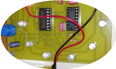
1. LED-Blinker: Die zwei Leuchtdioden blinken abwechselnd insgesamt 60 Mal in einer Minute.
