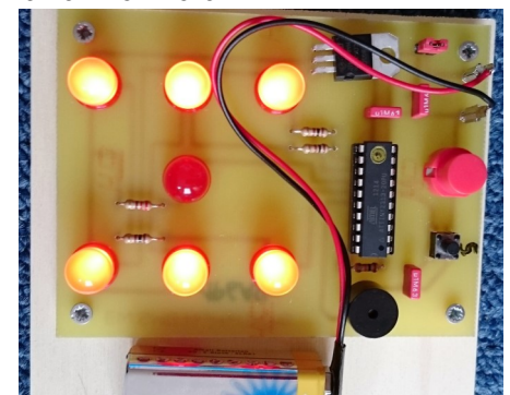
5. Elektronischer Würfel: Er kann bis sechs zählen wie ein normaler Würfel. Damit eignet er sich sehr gut zum Spielen von Würfelspielen.
