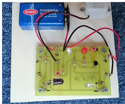
2. Lichtschranke mit Summer: Wenn etwas zwischen der Leuchtdiode und dem Fotowiderstand ist, gibt es ein lautes und nerviges Summen.
